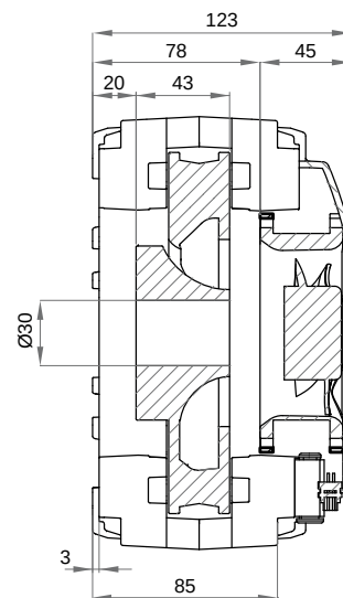
SEZIONE A-A
