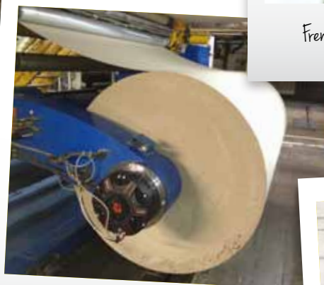
Freno Extreme su svolgitore Extreme brake on unwinder
